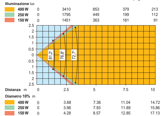
CP COLOR - Con filtro ovalizzatore opzionale (asse X)
