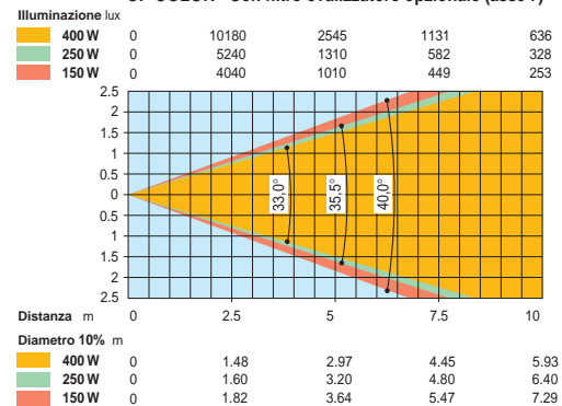
CP COLOR - Con filtro ovalizzatore opzionale (asse Y)
