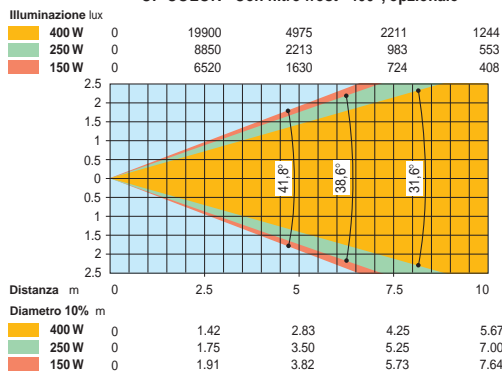
CP COLOR - Con filtro frost "400", opzionale
