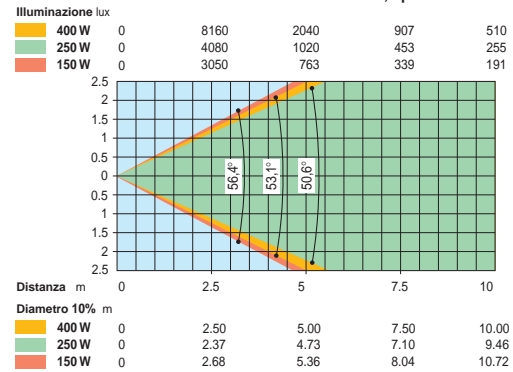
CP COLOR - Con filtro diffusore Ø 205 mm, opzionale
