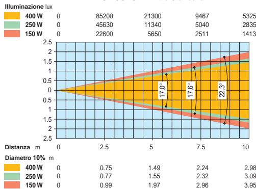
CP COLOR - Con filtro frost "C", opzionale
